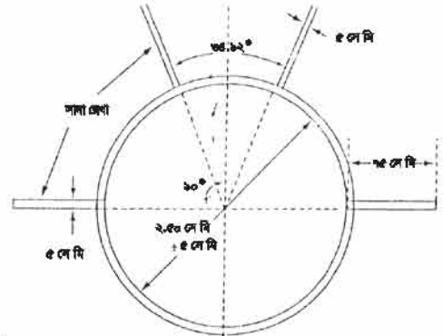
চাকতির সার্কেল ও স্টেটর
