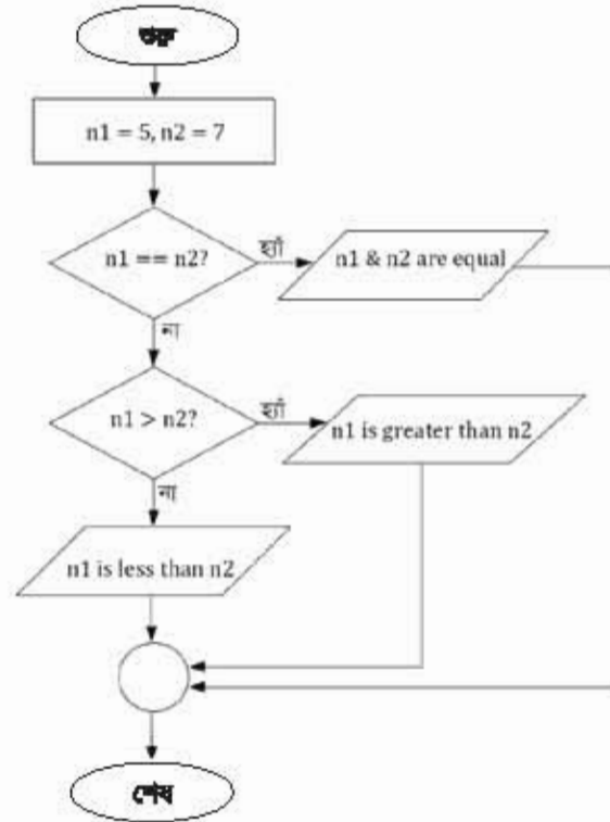
চিত্র 5.8: দুটি সংখ্যার মধ্যে তুলনা করার ফ্লোচার্ট
