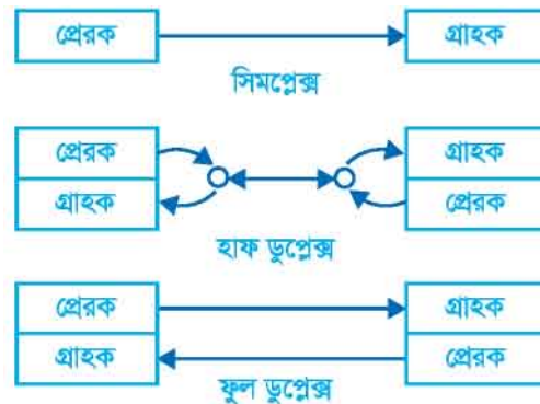
চিত্র 2.4: সিমপ্লেক্স, হাফ ডুপ্লেক্স এবং ফুল ডুপ্লেক্স
