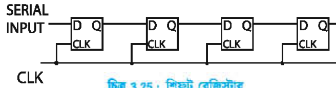
চিত্র 3.25 : শিফট রেজিস্টার
