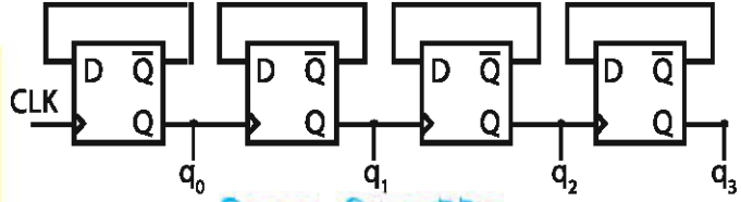
চিত্র 3.26 : রিপল কাউন্টার
